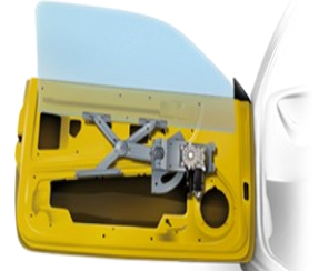
FENSTERHEBER MIT SCHERENSYSTEM
